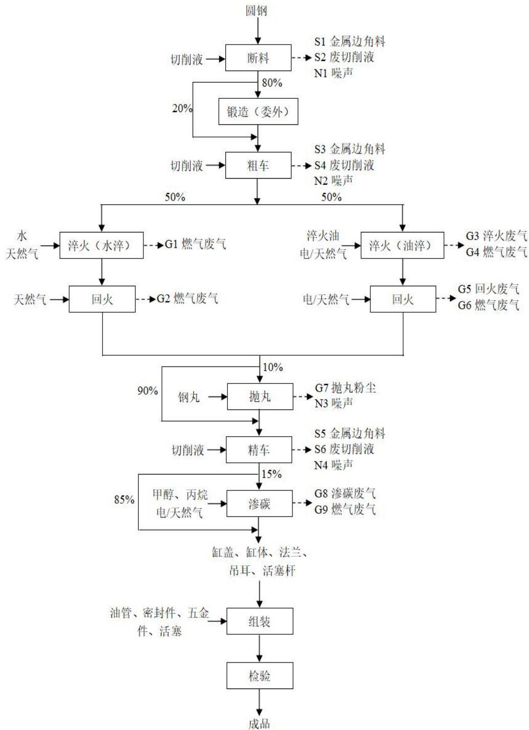
图 2-2 挖掘机油缸生产工艺流程图
