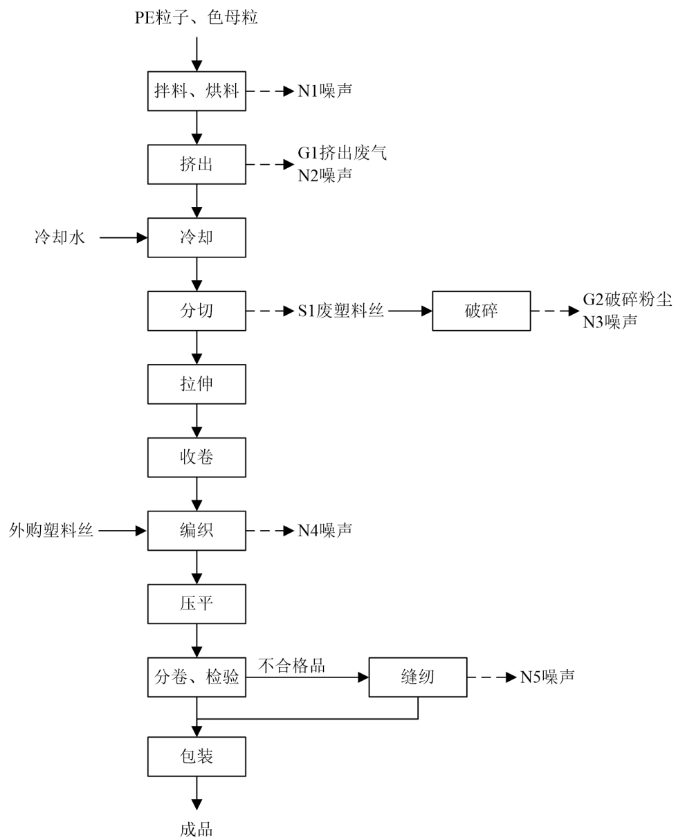
图 2-2 塑料遮阳网生产工艺流程图
