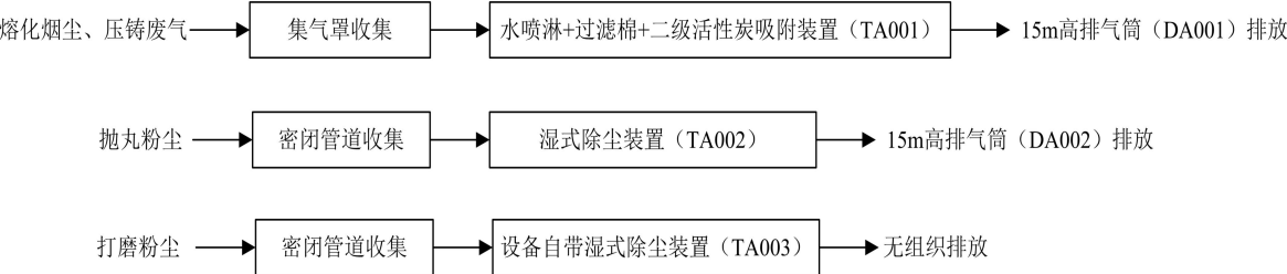
图 4-1 废气收集及处理工艺示意图
