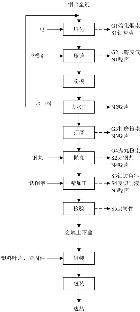
图 2-2 风叶轮生产工艺流程图
